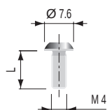
TORX T15
